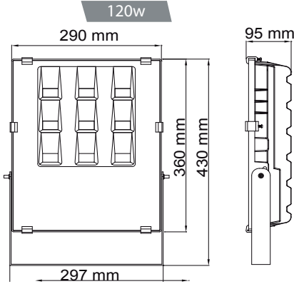
Peso = 5.1 kg
